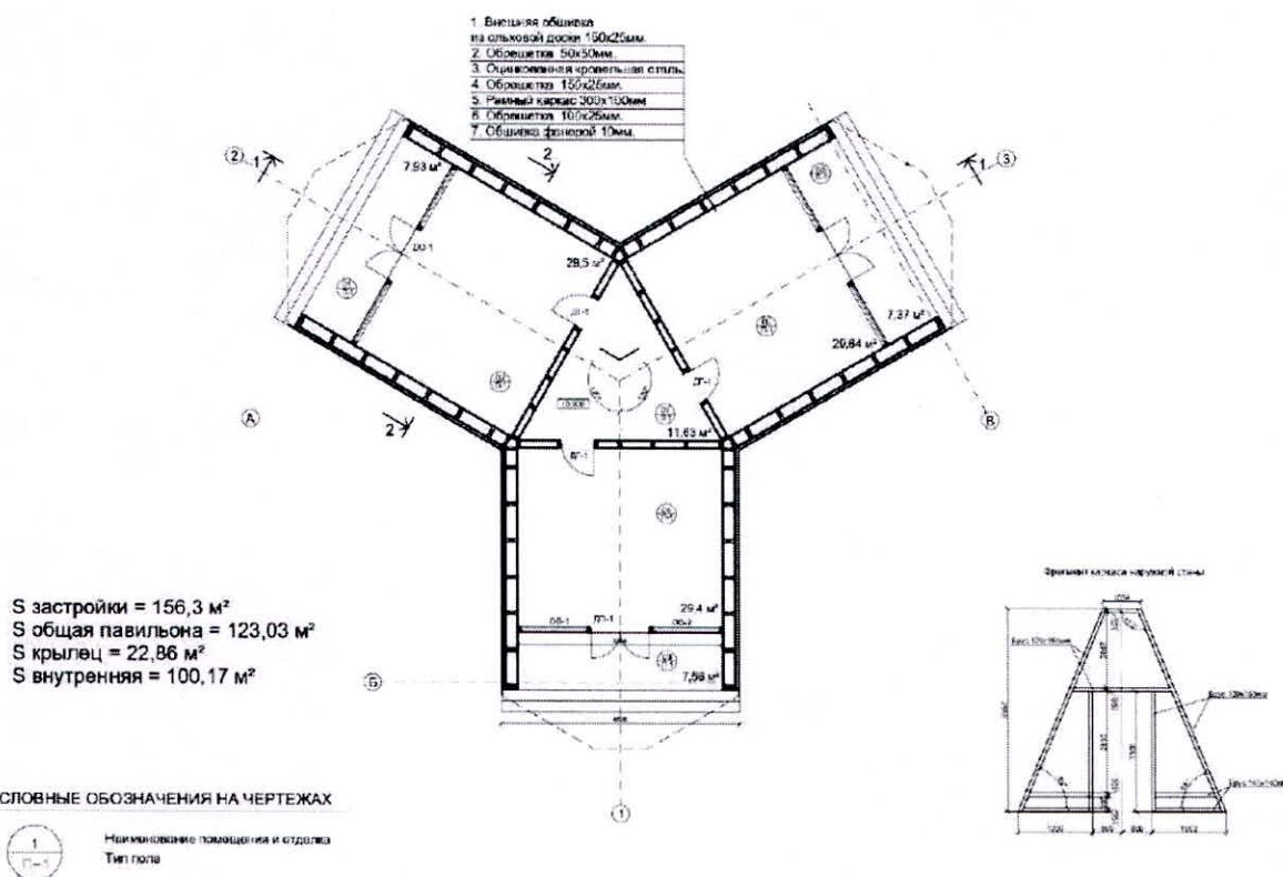
План паркового павильона "Трилистник"
